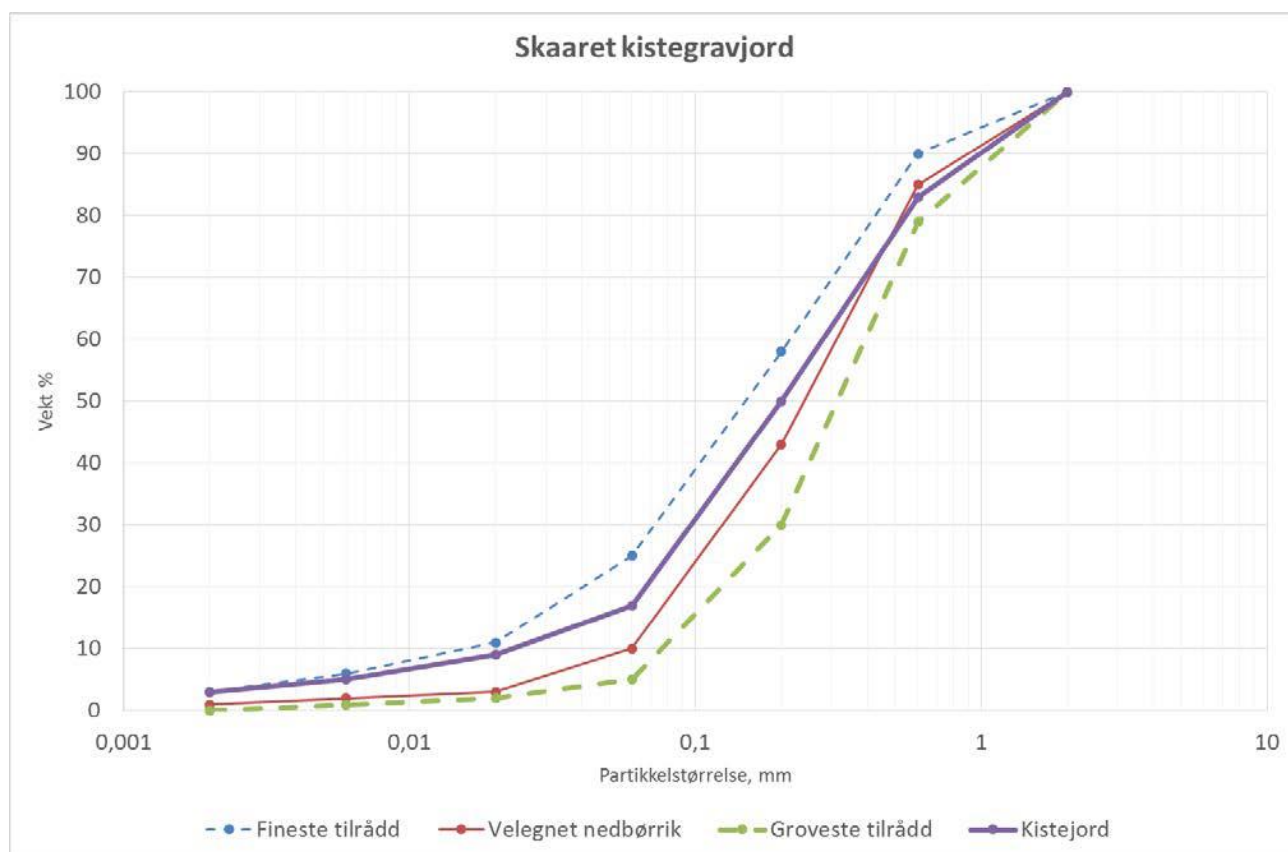
Figur 1. Kornfordelingskurve for Skaaret kistegravjord i forhold til anbefalt tekstur
